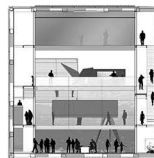
CORTE E3
