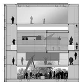
CORTE D1
